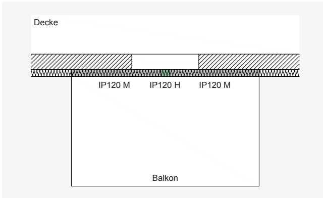
ISOPRO® 120 H – Ausragender Balkon mit planmäßig auftretenden Horizontalkräften
