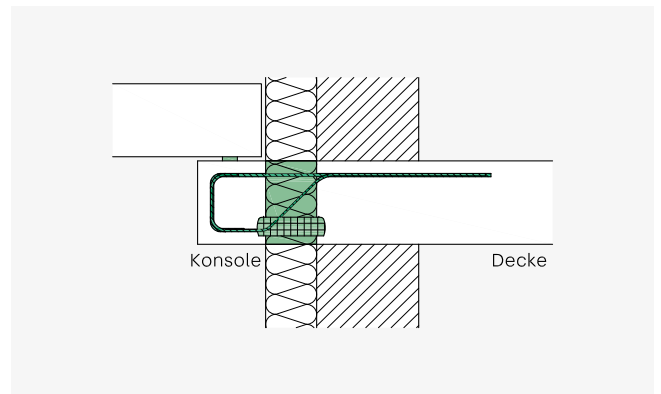
ISOPRO® 120 O - Konsole als Auflager für ein Fertigteilenelement, Auflage mit Zentrierlager
